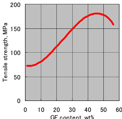
Fig.1 Tensile strength
