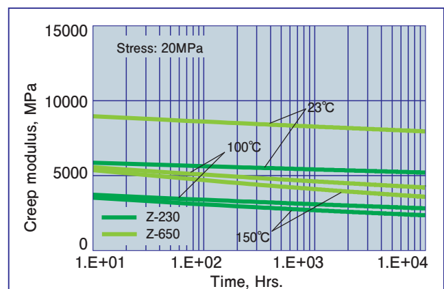
Fig.4.16 曲げクリープ弾性率の温度依存性 (スーパータフグレード) Flexural creep modulus of tough "Z" grades affected by temperature
