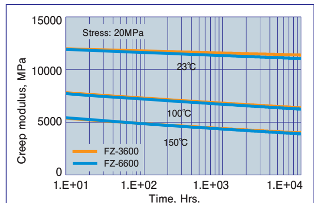
Fig.4.15 曲げクリープ弾性率の温度依存性 (フィラーグレード) Flexural creep modulus of GF/filler grades affected by temperature
